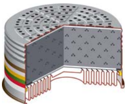
Dräger Filter Rd91: Schnittzeichnung
